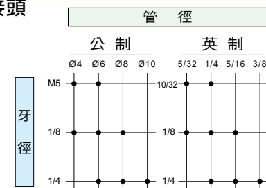
QVAH 開關螺牙接管
