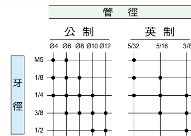
QSU L型迴轉接頭
