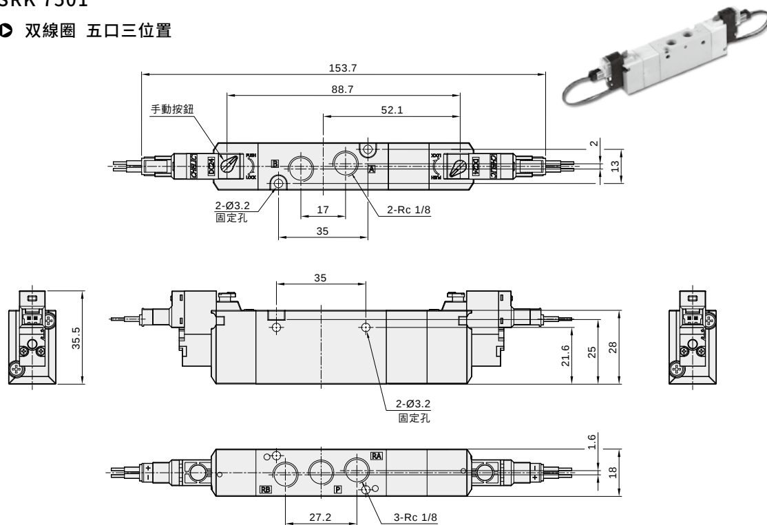
SRK 7301 (中閉型) N.C.
