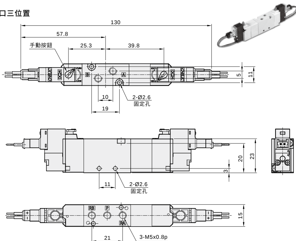
SRK 5(3)0M5 (中閉型) N.C.
