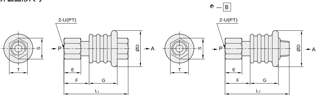
◎ 外觀圖形尺寸
