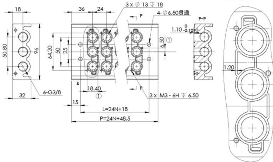
局部视图
