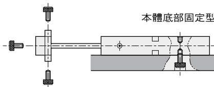
滑塊可由三方向固定
