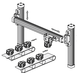
● 搬運作業
