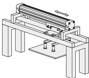
● 水平移載
