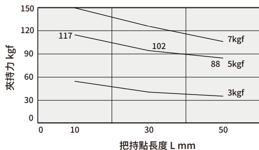
HCW、HCWL 60 - OPEN
