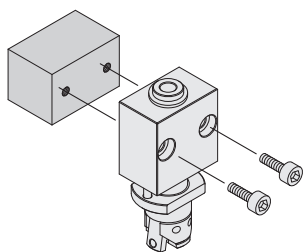
方形後座型固定方式
