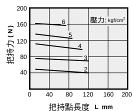
HDT 25100 HDT 25120
