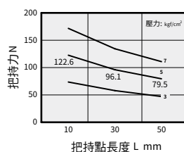
HDW 20 - OPEN
