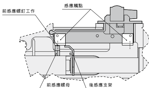
(活塞在前端狀態)
