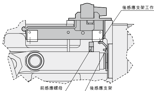
(活塞在後端狀態)
