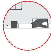
◉ 金屬刮塵環
