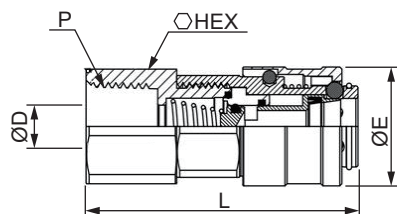
QC1SF:C式快接母內牙型
