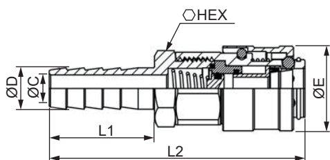
QC1SH:C式快速母插芯型
