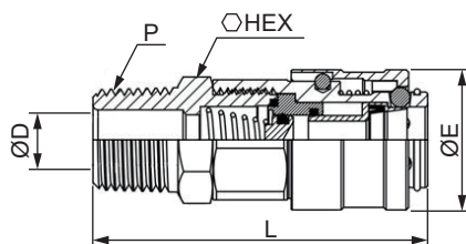
QC1SM:C式快接母外牙型
