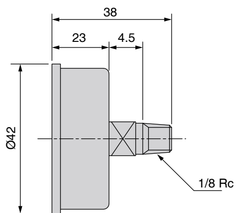
外觀圖形尺寸
