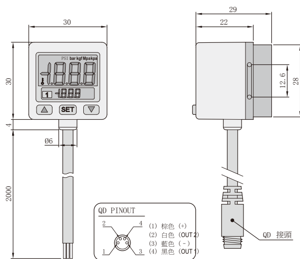
► 外觀尺寸圖
